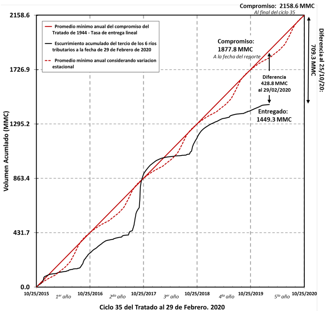
Figura 1. Volumen acumulado del agua asignada a los Estados Unidos del Ciclo 35 (del 25/Oct/2015 al 31/Ene/2020) proveniente de los seis afluentes mexicanos de acuerdo con lo establecido en el Tratado de 1944.
